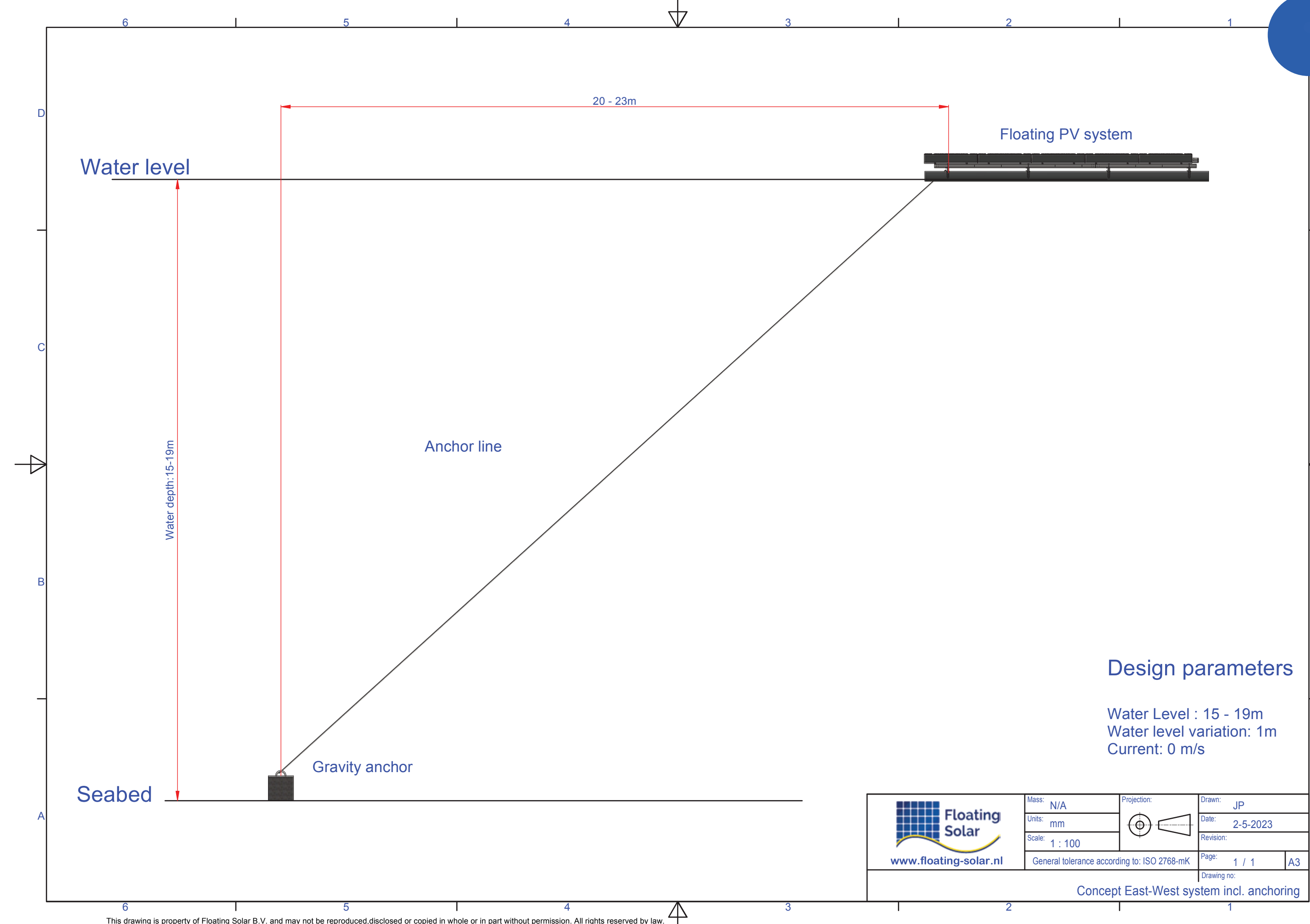
Verankering PV-systeem
